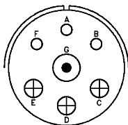
DISPOSICIÓN 24-16 TAMAÑO CONTACTOS 1/8 , 3/12 , 3/16 RANGO DE SEVICIO A,B,F,G=D ; C,D,E=A
