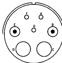
32-10 2/4 , 2/8 , 3/16 A,F=E ; B,E=D ; C,D=A ; G=B
