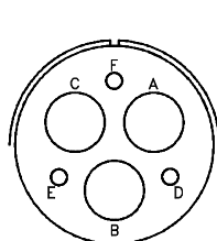
DISPOSICIÓN 28-22 TAMAÑO CONTACTOS 3/4 , 3/16 RANGO DE SERVICIO D
